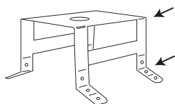
UG-beslaget är lätt att böja/forma så att det passar runda eller plana kanaler. The UG-bracket can easily be bent or shaped to fit circular or rectangular duct.
