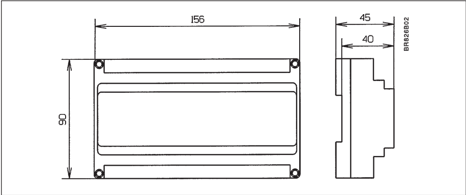
Fig. 15 - Dimensions
