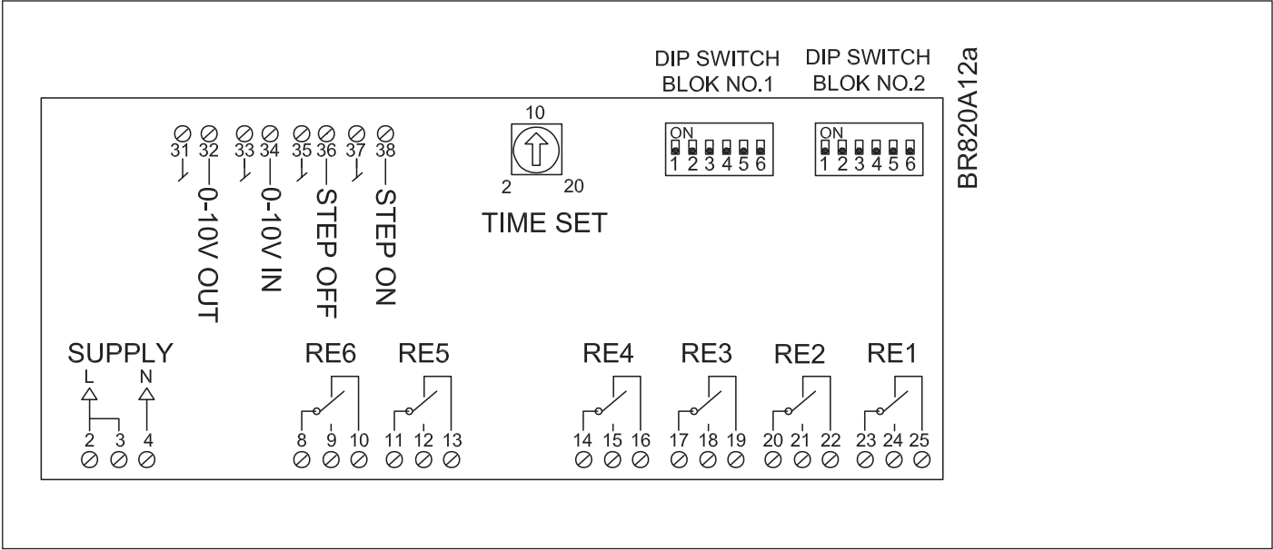
Fig. 1 - Wiring diagram
